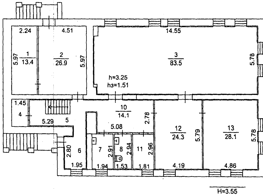
План цокольного этажа
