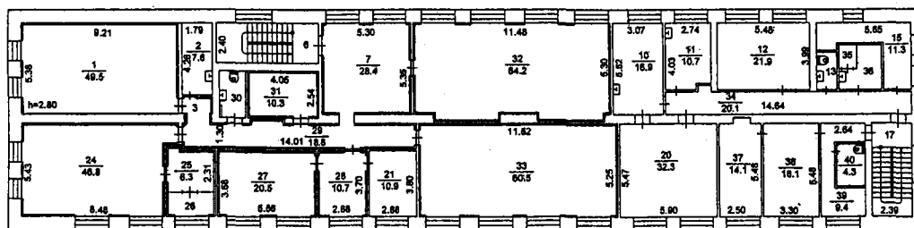
План 2 этажа
