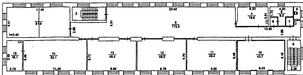
План 4 этажа
